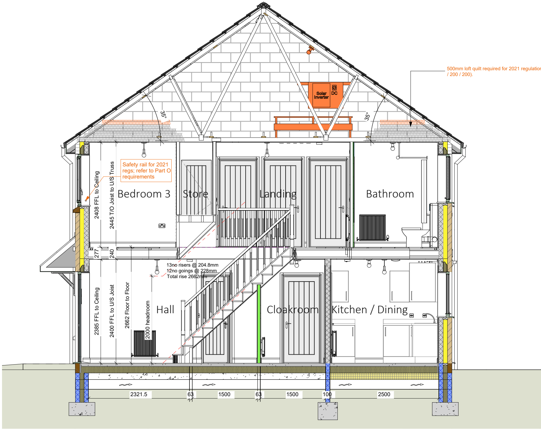
B Section B - B 1 : 50
